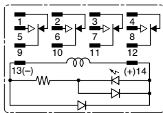
4PDT (RY4)
